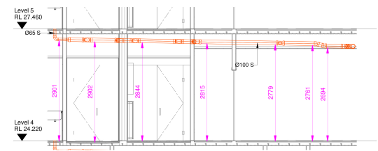
S8 SECTION L4-S8 H412 1:50
